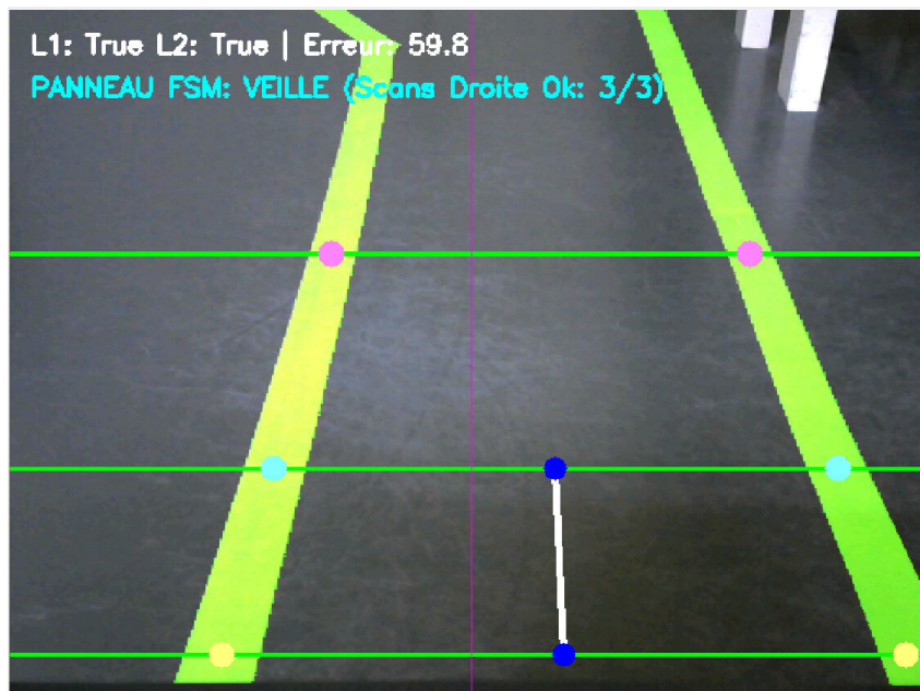
FIGURE 1 – Représentation géométrique des horizons d'analyse ( L1, L2, L3 ) et fenêtrage de la route dans le plan image.
