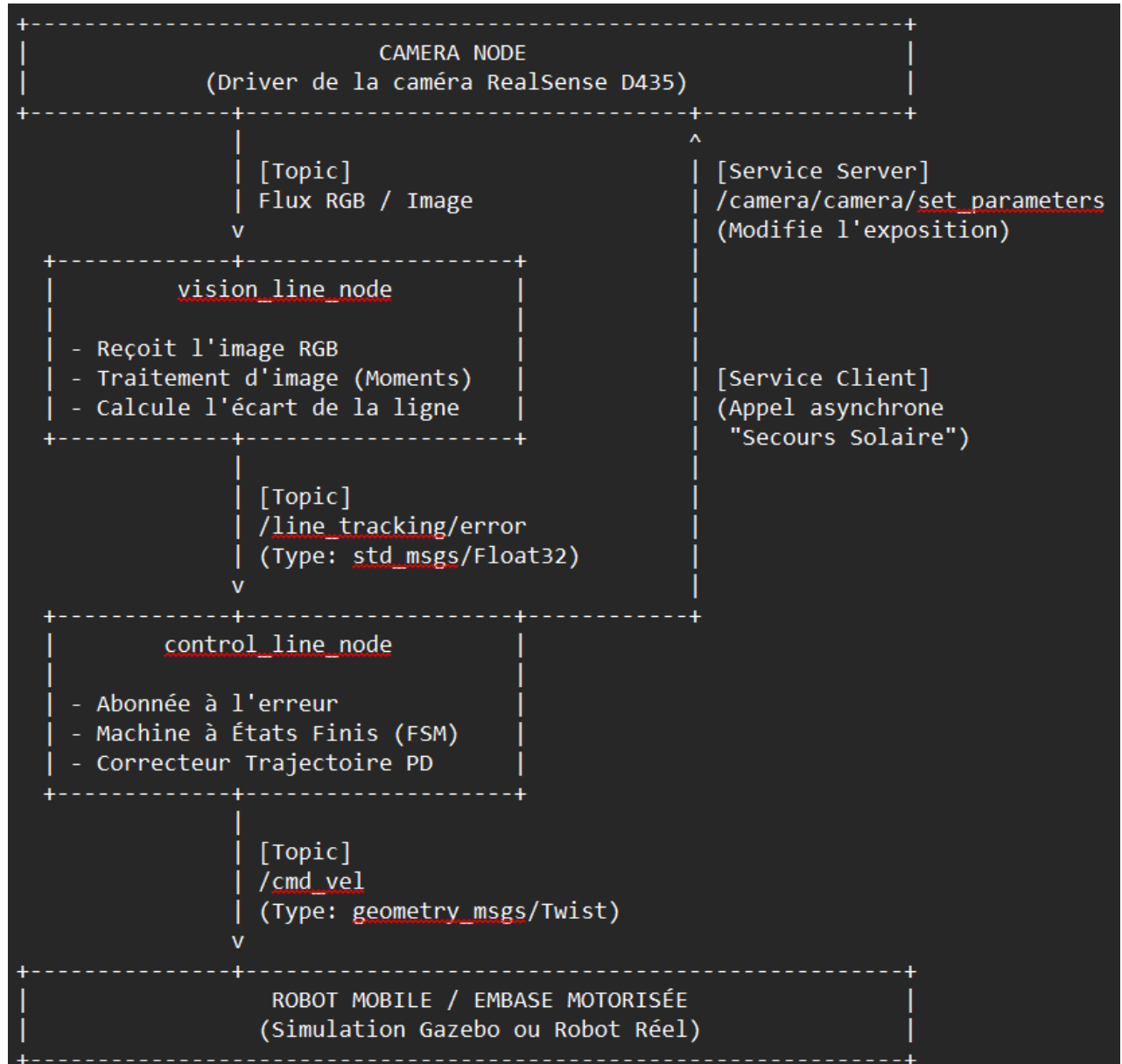
FIGURE 2 – Architecture logicielle, interconnexions par Topics et Services entre la caméra, le nœud de vision et le nœud de commande cinématique.
